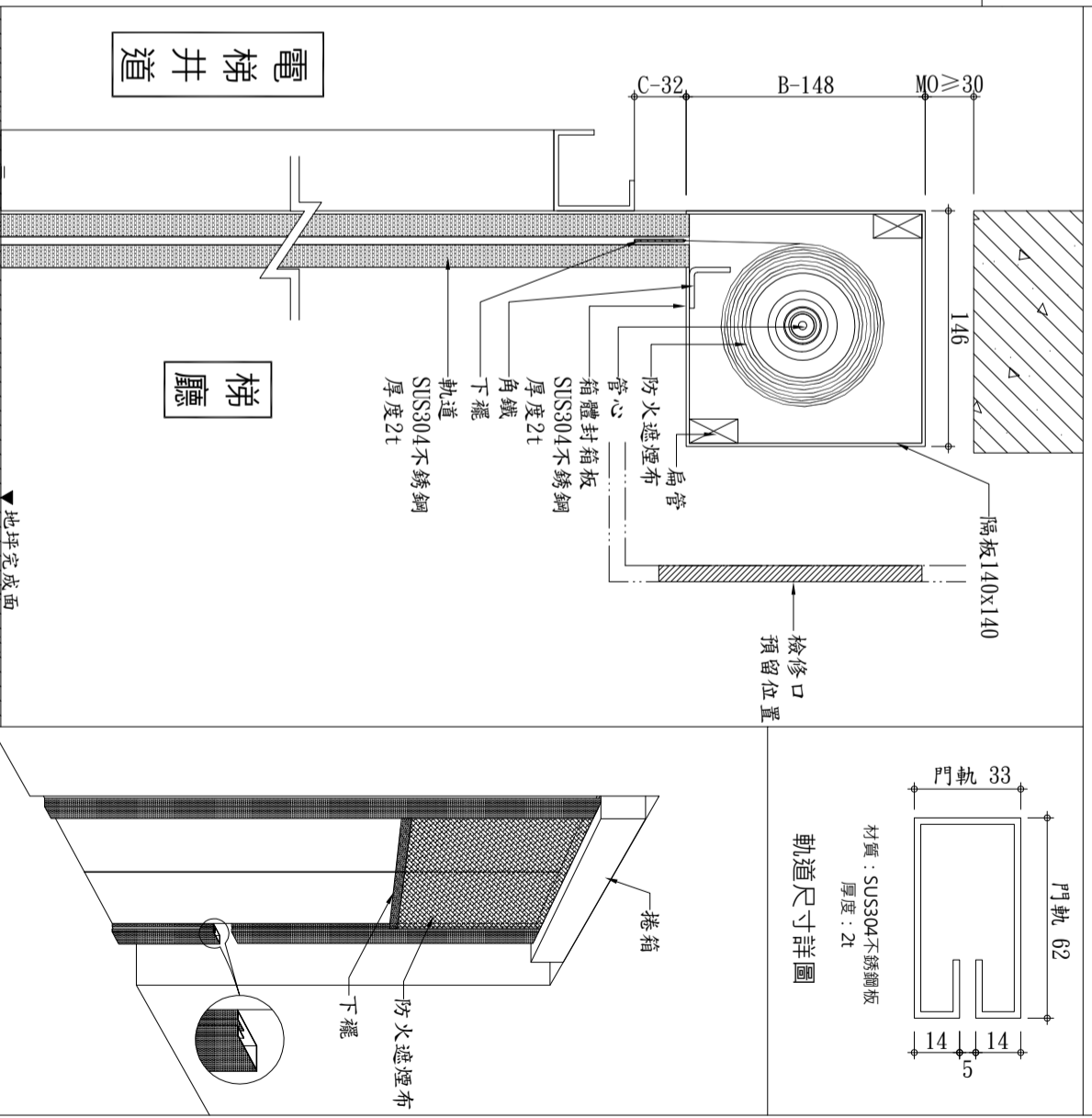
機箱剖面含介面說明示意詳圖
