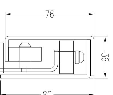
上門軌詳圖
