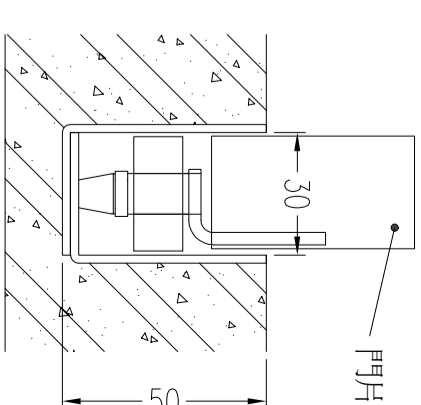
上門軌詳圖
